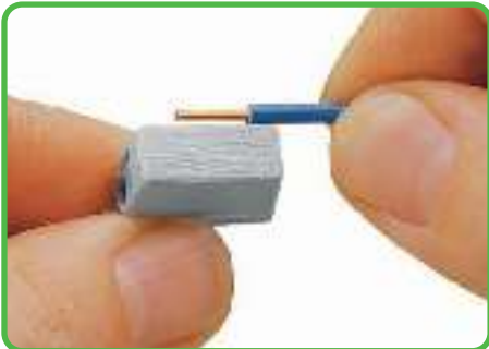
Изоляцию проводника снять на длине 9 - 11 мм
